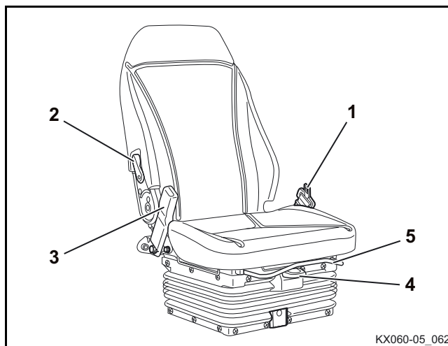
Vzduchem odpružené sedadlo (na přání)
