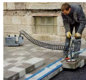
Ruční vakuové manipulační zařízení MICROJUMBO MJ
