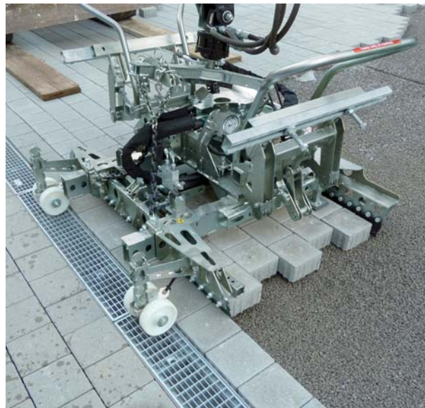
HVZ-ECO Hydraulické pokládací kleště
