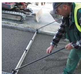
TELEPLAN TP Ruční stahovací systém
