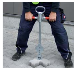
Vytahovací kladivo SZH
